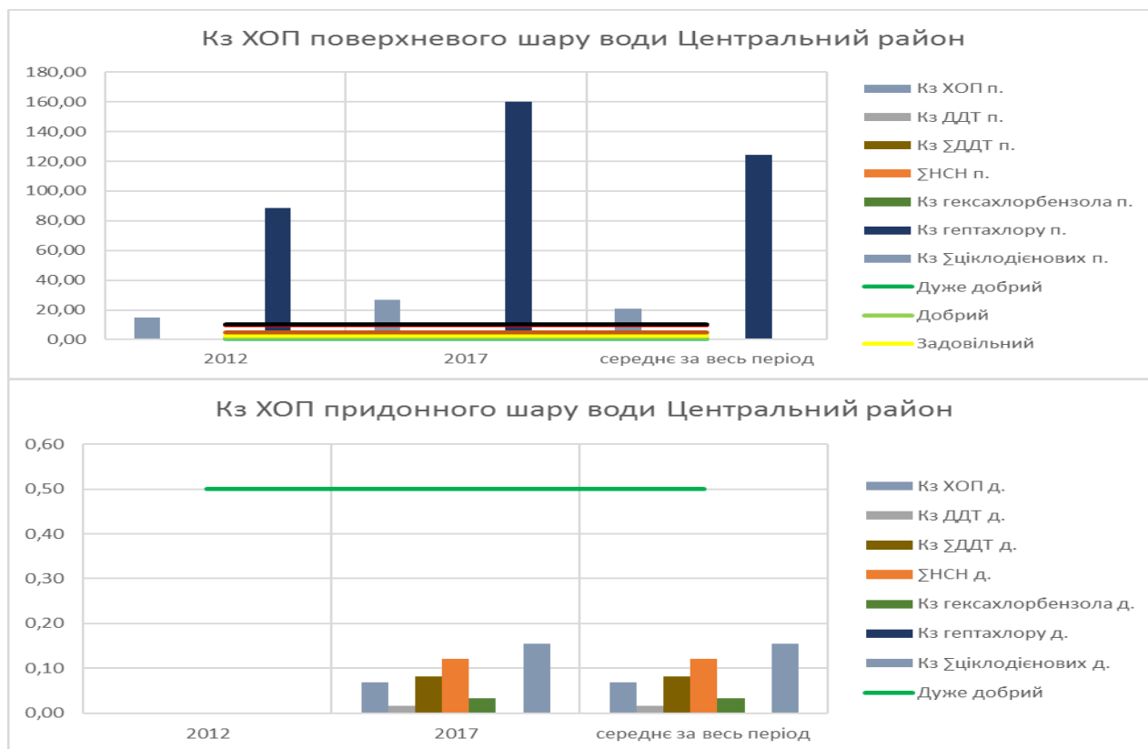
Рисунок 1.46 – Кз ХОП морської води центрального району з 2012 по 2017 роки
