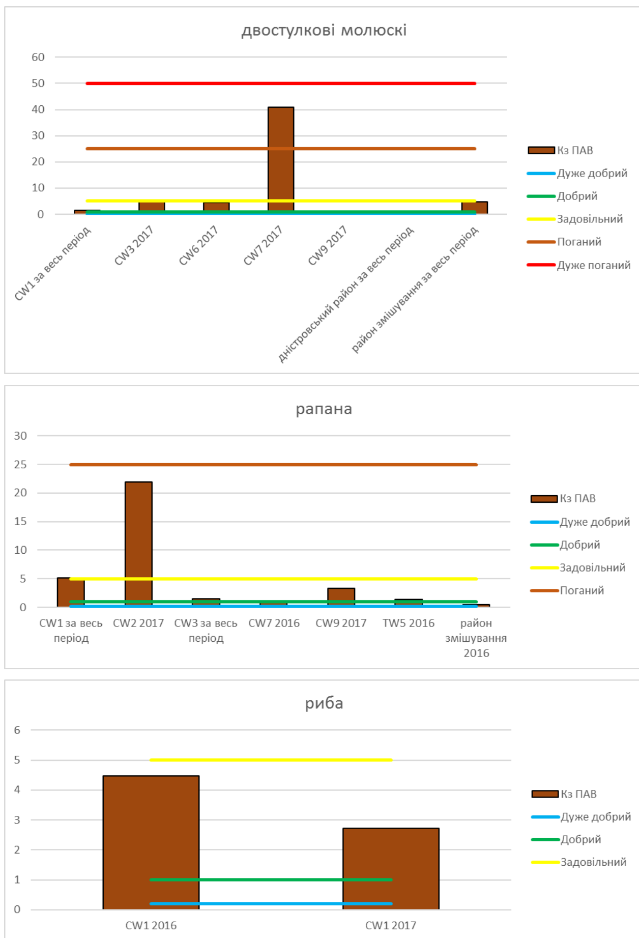
Рисунок 3.3 – Середні Кз ПАВ двостулкових молюсків, рапана, риби
