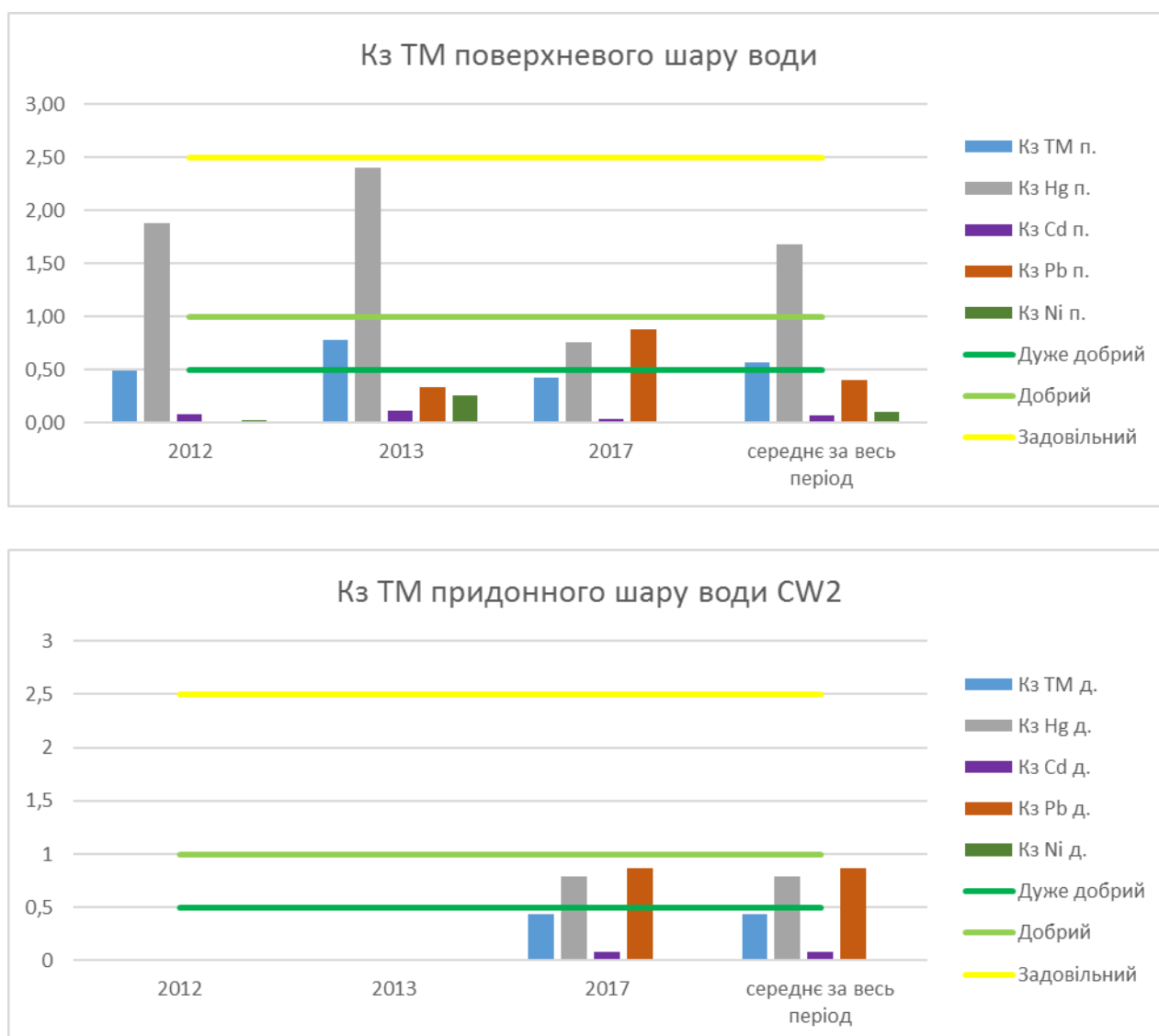
Рисунок 1.14 – Кз ТМ морської води у водному тілі CW2
