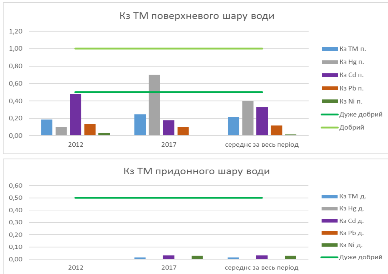
Рисунок 1.45 – Кз ТМ морської води центрального району
