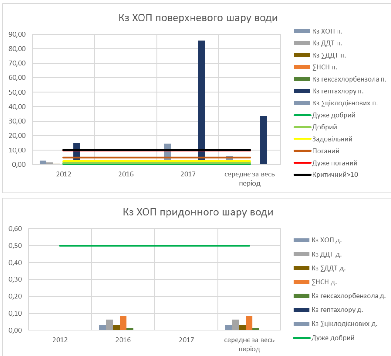
Рисунок 1.40 – Кз ХОП морської води Дніпро – Бузького району з 2012 по 2017 роки
