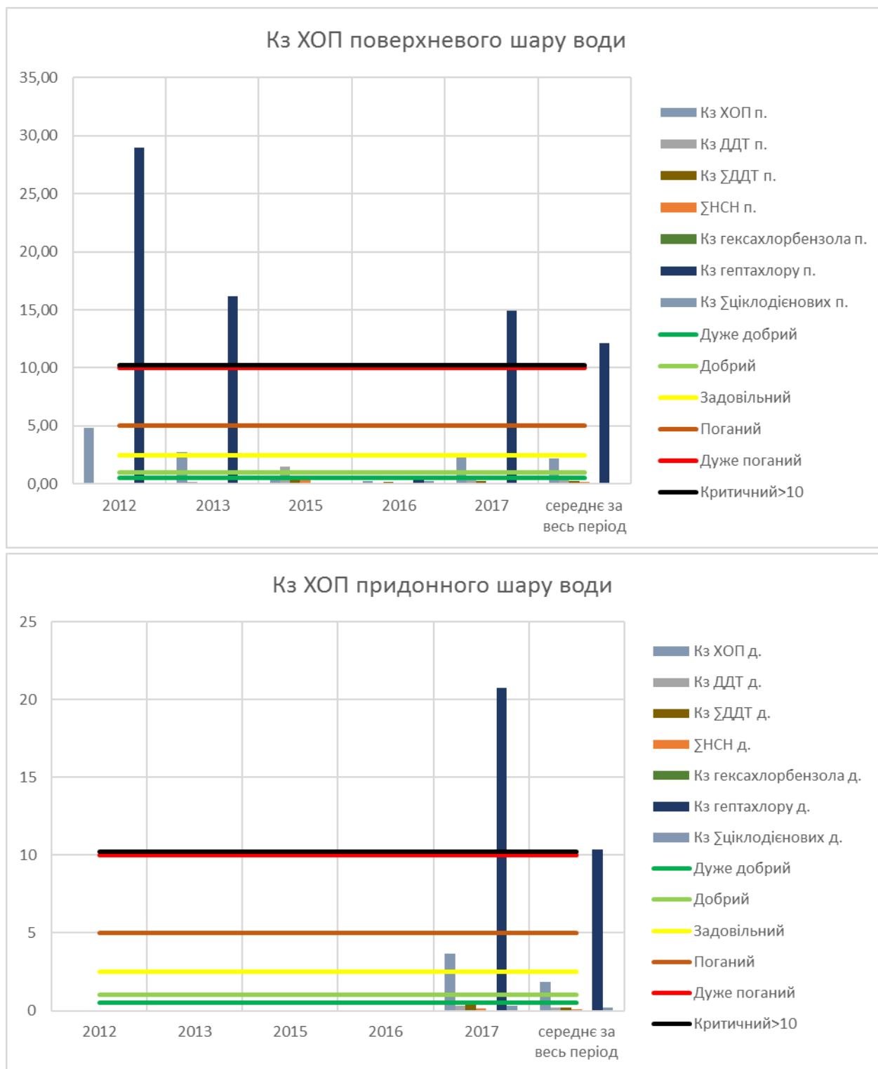
Рисунок 1.11 – Кз ХОП морської води в Дунайському районі
