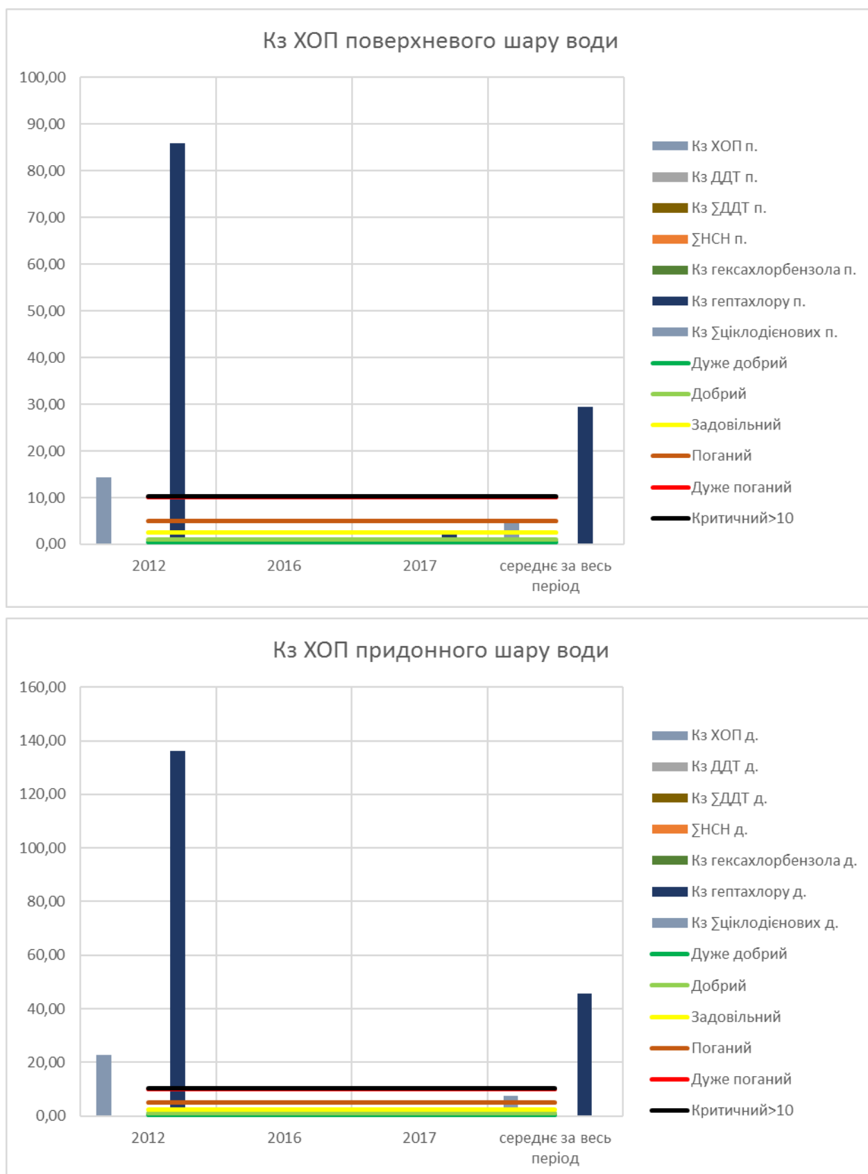
Рисунок 1.43 – Кз ХОП морської води району змішування з 2012 по 2017 роки
