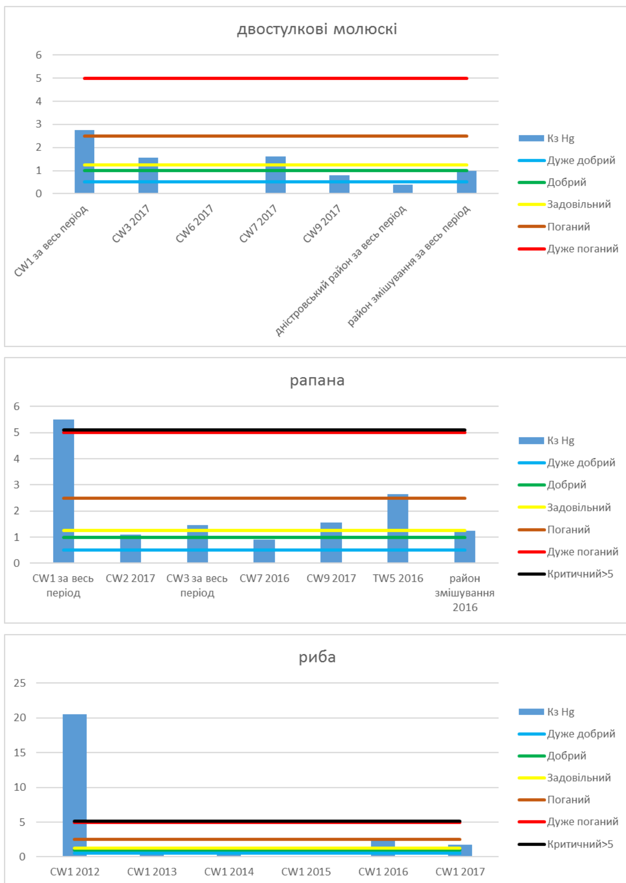
Рисунок 3.1 – Середні Кз ТМ двостулкових молюсків, рапана, риби по районах та водних тілах ПЗЧМ
