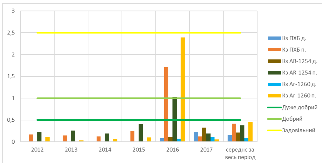
Рисунок 1.8 – Кз ПХБ морської води в водному тілі TW5 з 2012 по 2017 роки
