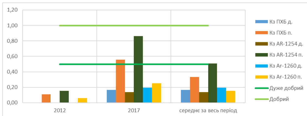
Рисунок 1.38 – Кз ПХБ морської води в водному тілі CW9
