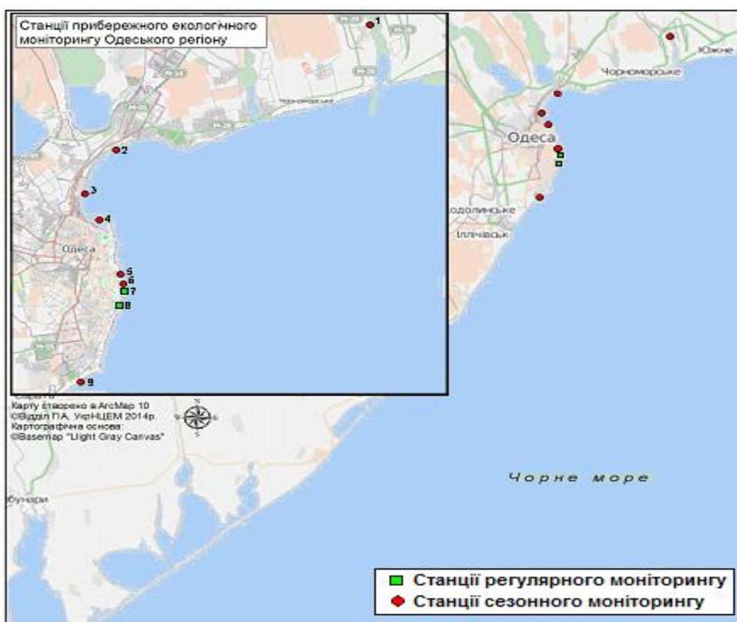
Рисунок 4.1 – Схема розташування станцій гідробіологічного моніторингу Одеського регіону у 2017 році
