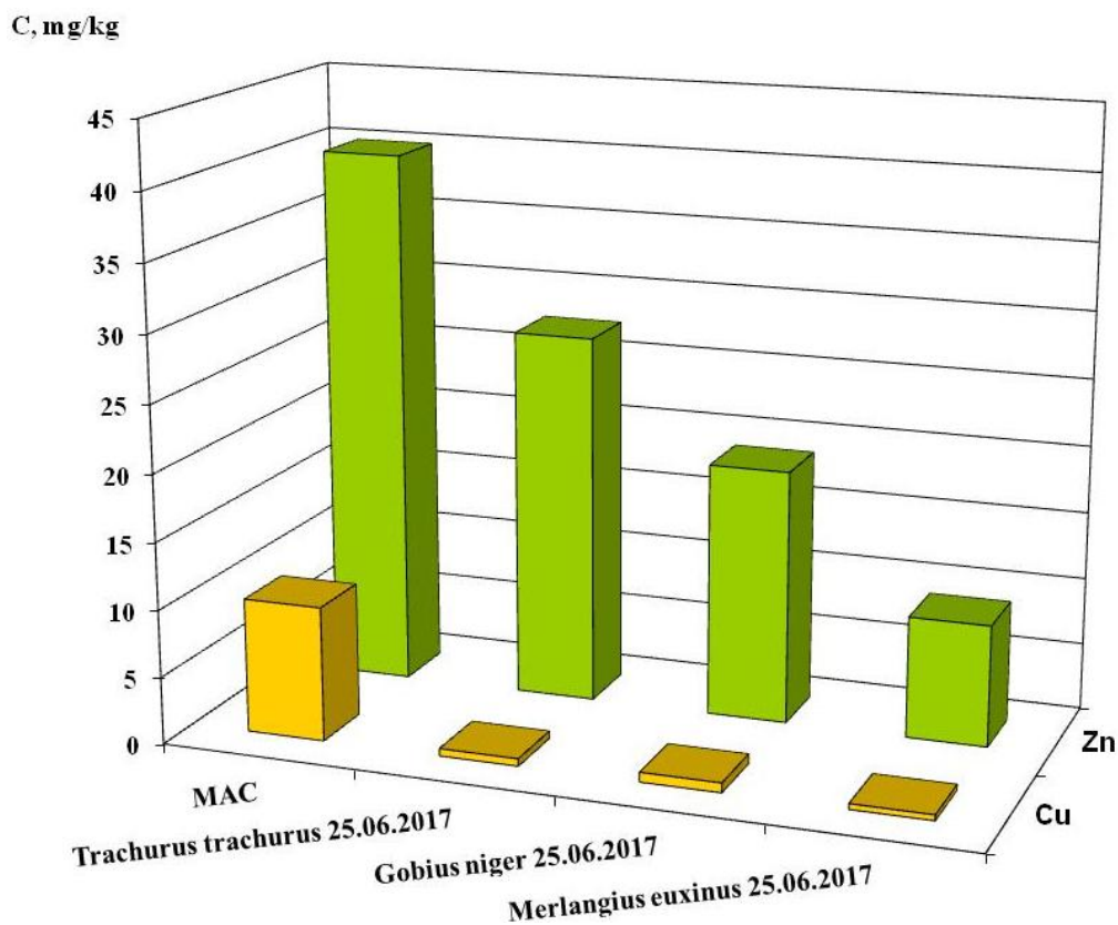
Рисунок 3.102 – Концентрації токсичних металів (Cu, Zn) в тканинах риби (о. Зміїний)
