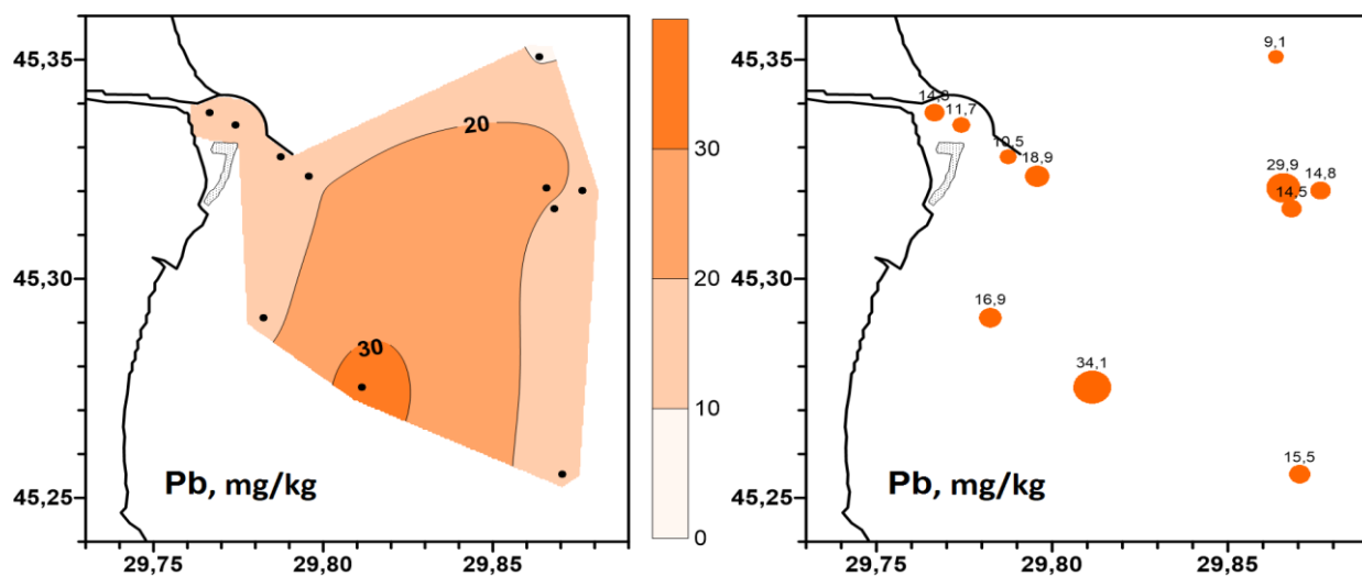
Рисунок 3.66 – Просторовий розподіл свинцю в д/в, мг/кг
