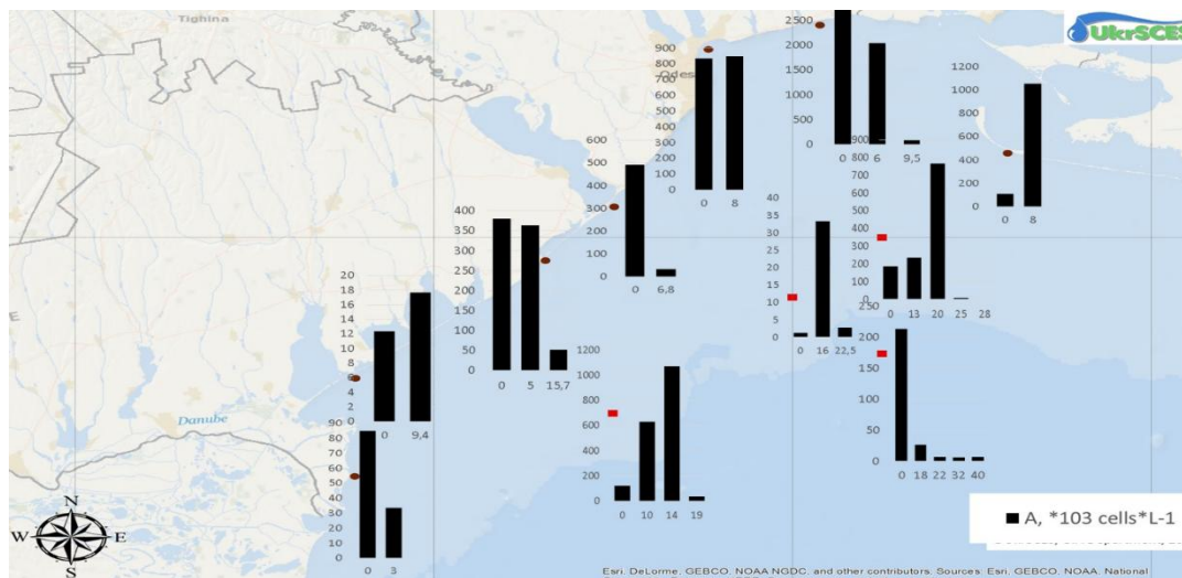
Рисунок 4.5 – Просторовий та вертикальний розподіл чисельності фітопланктону в українській частині шельфу Чорного моря в серпні 2017 р.
