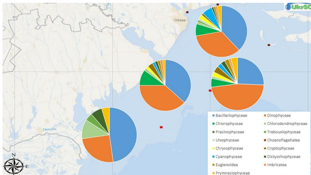
Рисунок 4.3 – Біорізноманіття фітопланктону в різних районах ПЗЧМ в серпні 2017 року
