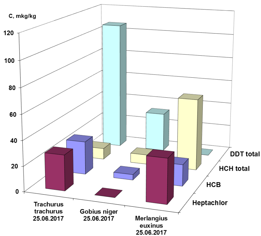
Рисунок 3.109 – Концентрації ХОП в тканинах риб (о. Зміїний)
