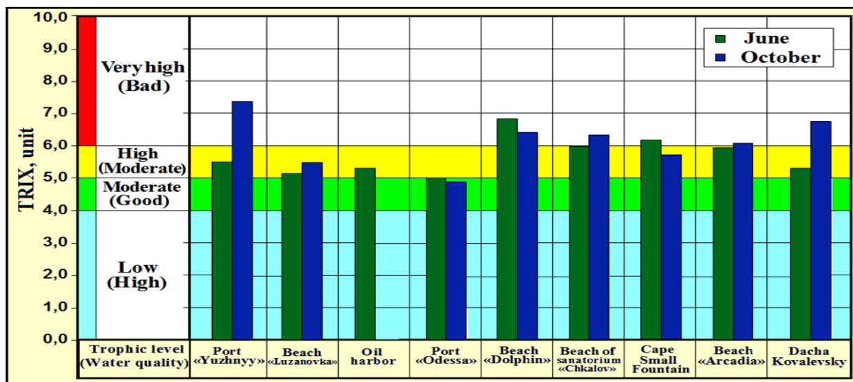
Рисунок 5.4 – Значення індексу трофності TRIX та якості прибережних вод Одеського регіону ПЗЧМ
