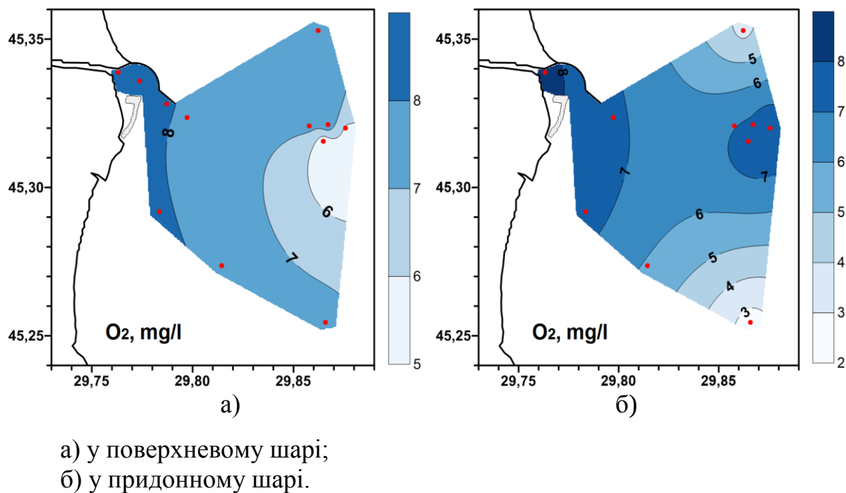
Рисунок 2.8 – Просторовий розподіл розчиненого у воді кисню (мг/л) на узмор'ї гирла Бистре у серпні 2017 року
