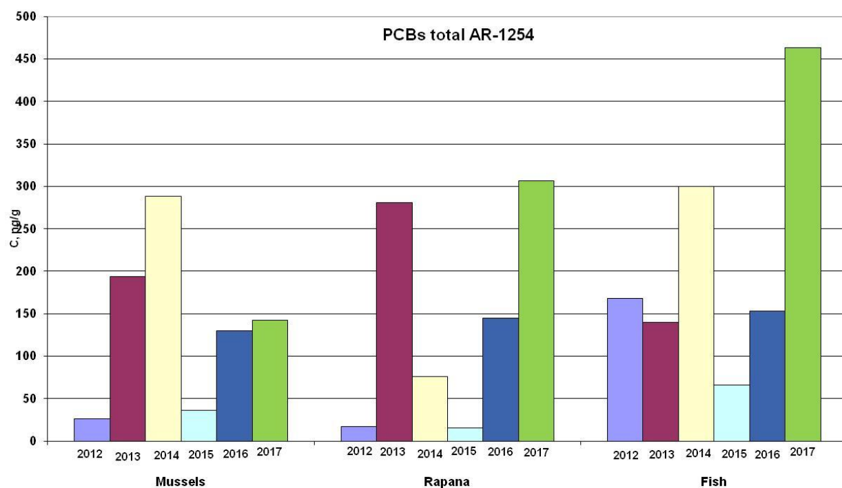
Рисунок 3.119 – Концентрації суми ПХБ (AR-1254) у тканинах мідій, рапанів та риб (о. Зміїний)
