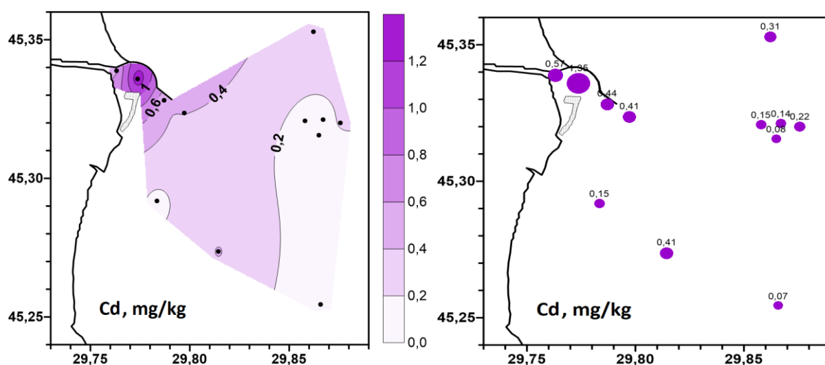
Рисунок 3.60 – Просторовий розподіл кадмію в д/в, мг/кг
