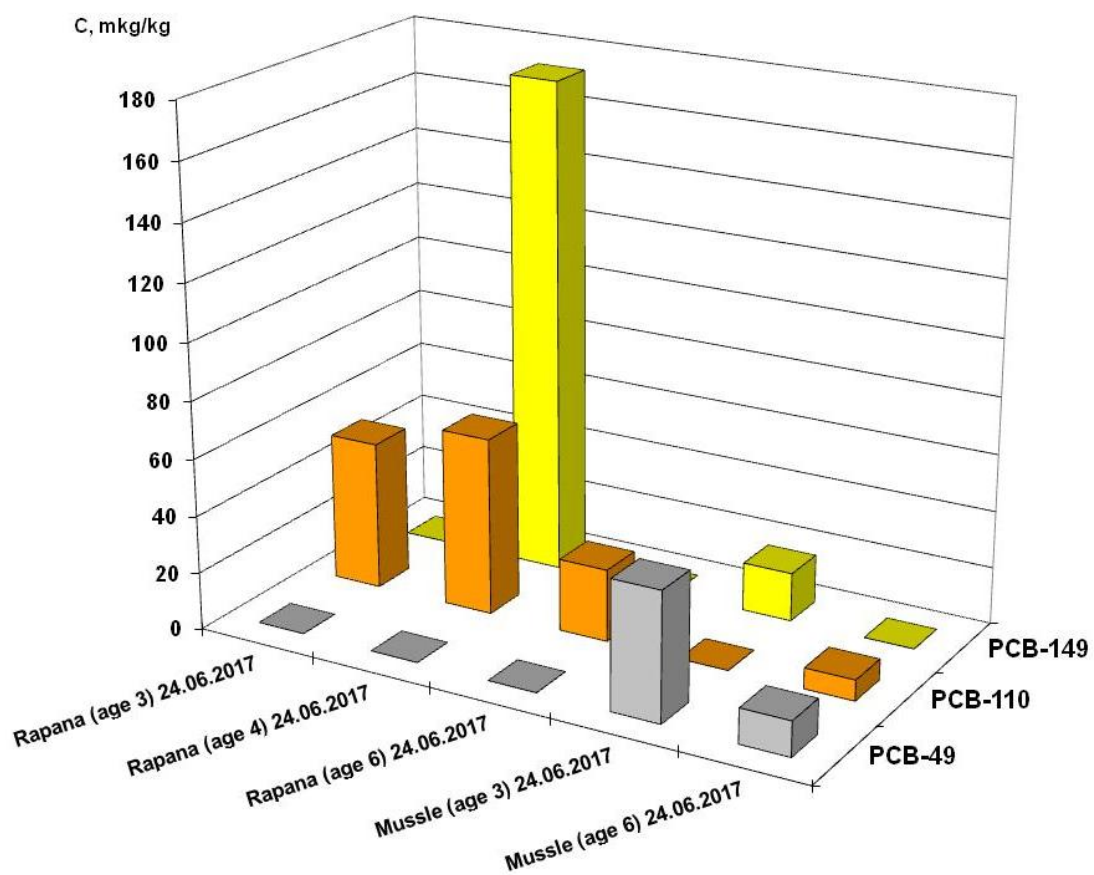
Рисунок 3.113 – Концентрації ПХБ (49, 110, 149) в тканинах мідій і рапани (о. Зміїний)
