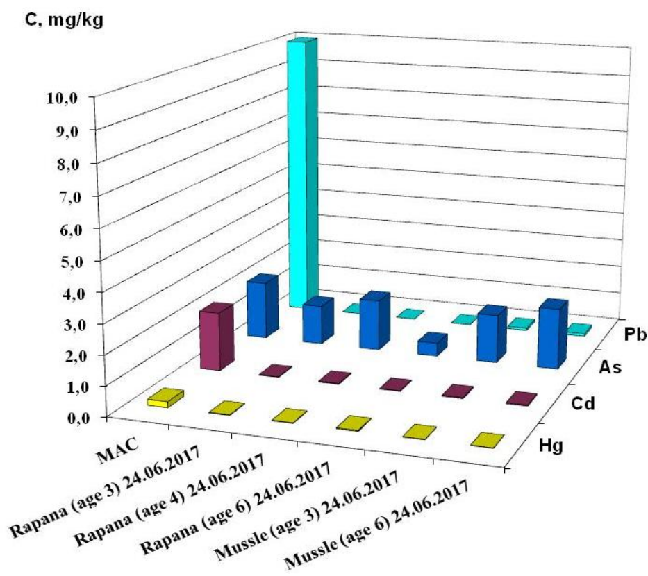
Рисунок 3.99 – Концентрації токсичних металів (Hg, Cd, As, Pb) в тканинах рапанів та мідій (о. Зміїний)
