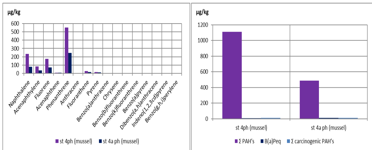
Рисунок 3.94 – Концентрації ПАВ у зразках біоти експедиції «NPMS-UA Phyllorhoga» (квітень)
