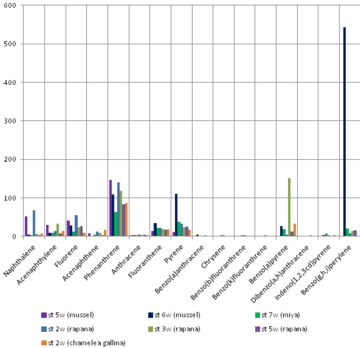
Рисунок 3.97 – Концентрації ПАВ у зразках біоти експедиції «NPMS-UA Water bodies» (серпень)
