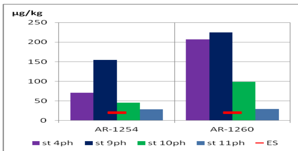
Рисунок 3.41 – Концентрація сум ПХБ в пробах д/в експедиції «NPMS-UA Phyllophora» (серпень)
