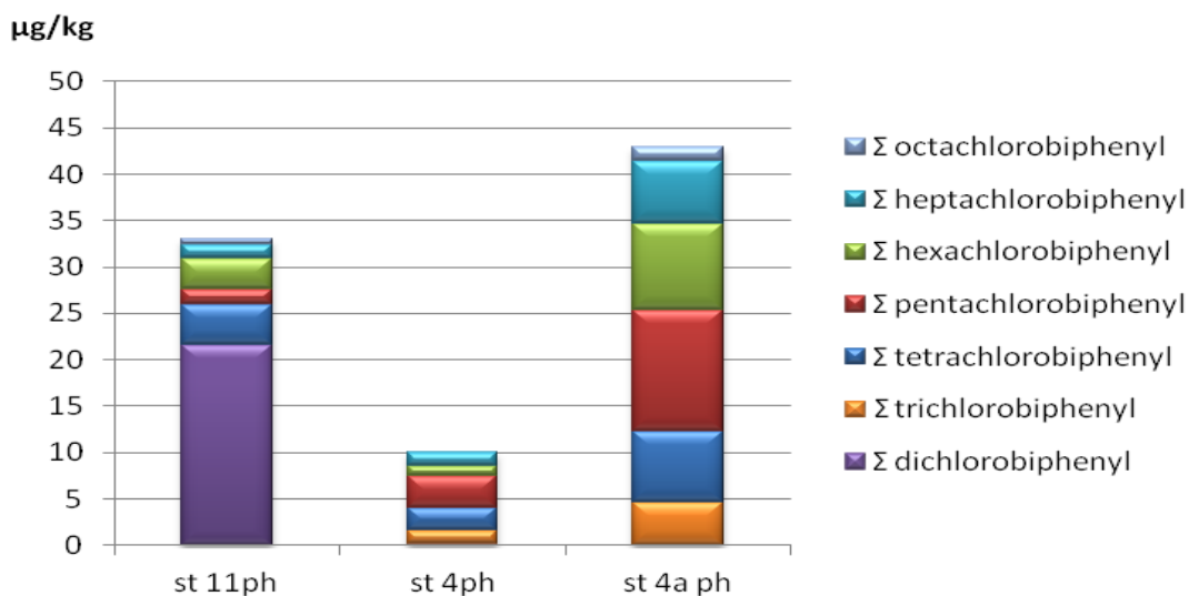
Рисунок 3.36 – Концентрації сум індивідуальних ПХБ з різним вмістом атомів хлору в пробах д/в експедиції «NPMS-UA Phyllophora» (квітень)
