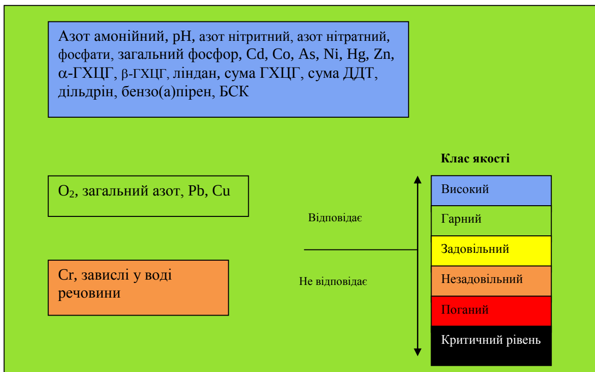
Рисунок 3.19 – Класи якості морської води експедиції «NPMS-UA Phyllophora» (серпень)
