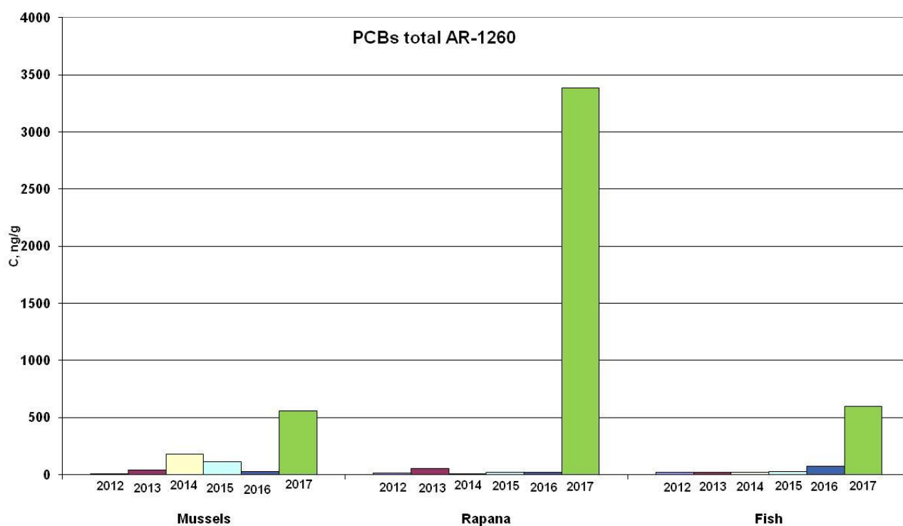
Рисунок 3.120 – Концентрації суми ПХБ (AR-1260) у тканинах мідій, рапанів та риб (о. Зміїний)
