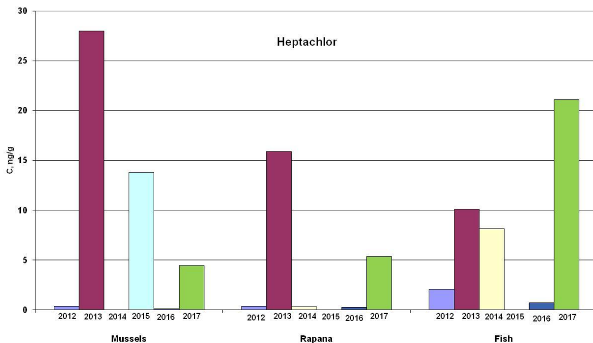
Рисунок 3.117 – Концентрації гептахлору у тканинах мідій, рапанів та риб (о. Зміїний)
