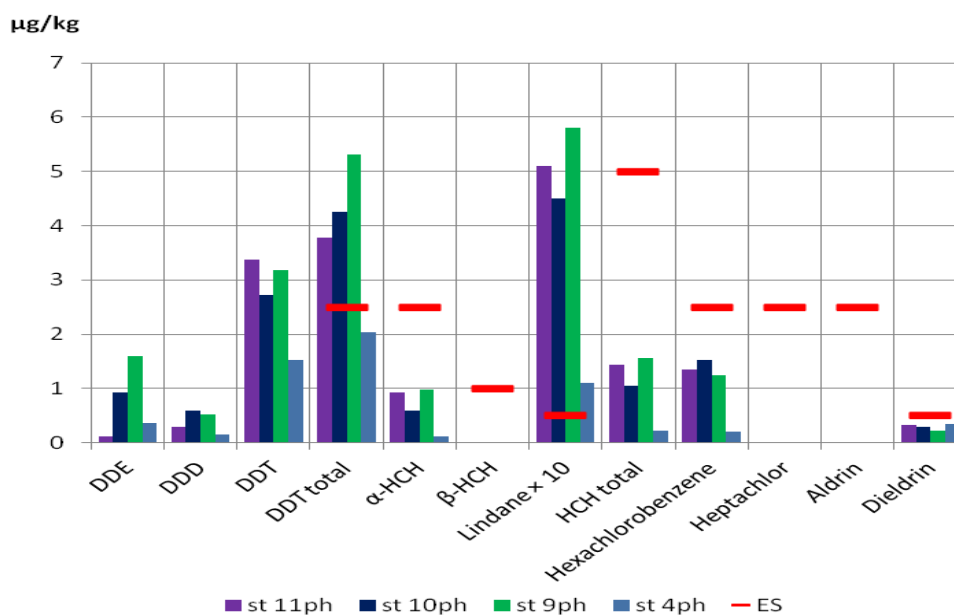
Рисунок 3.37 – Концентрації ХОП в д/в експедиції «NPMS-UA Phyllophora» (липень)
