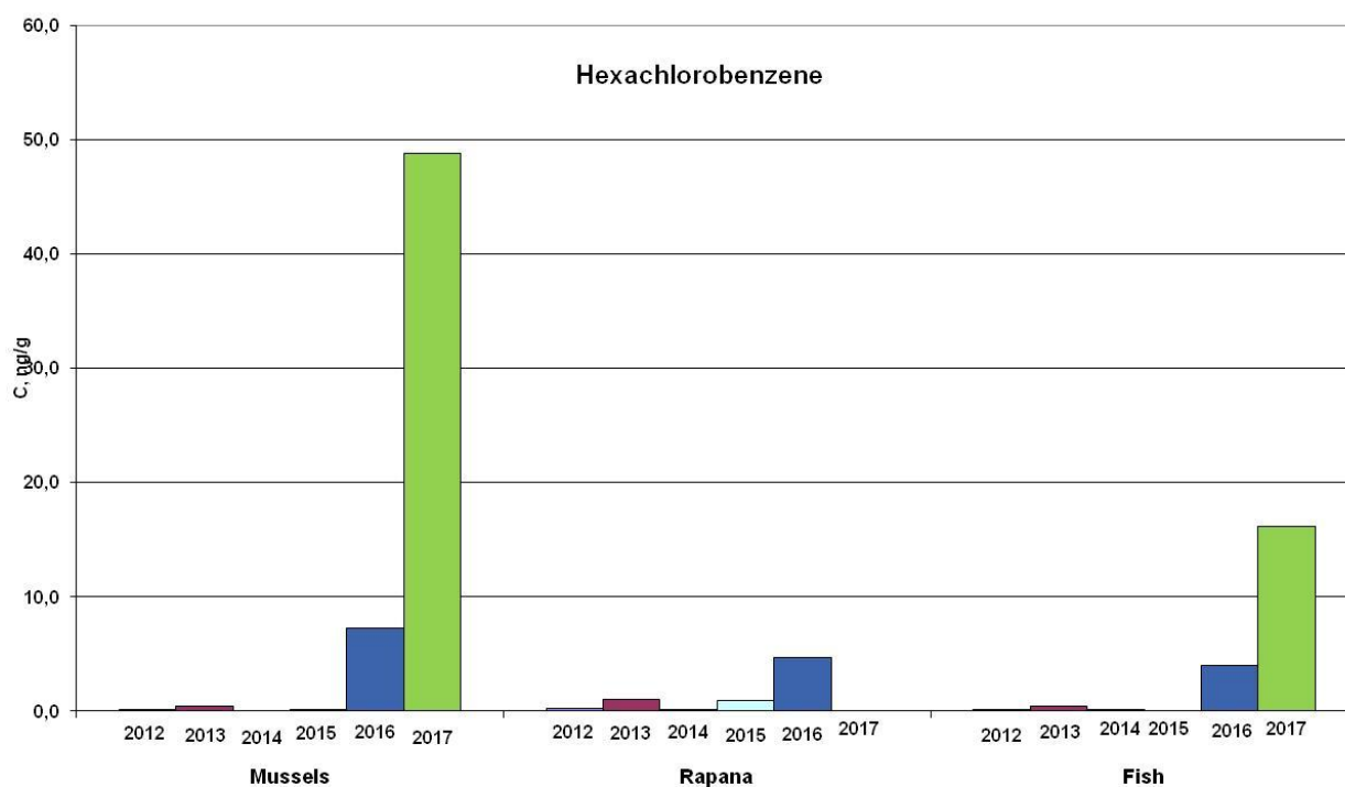
Рисунок 3.118 – Концентрації ГХБ у тканинах мідій, рапанів та риб (о. Зміїний)
