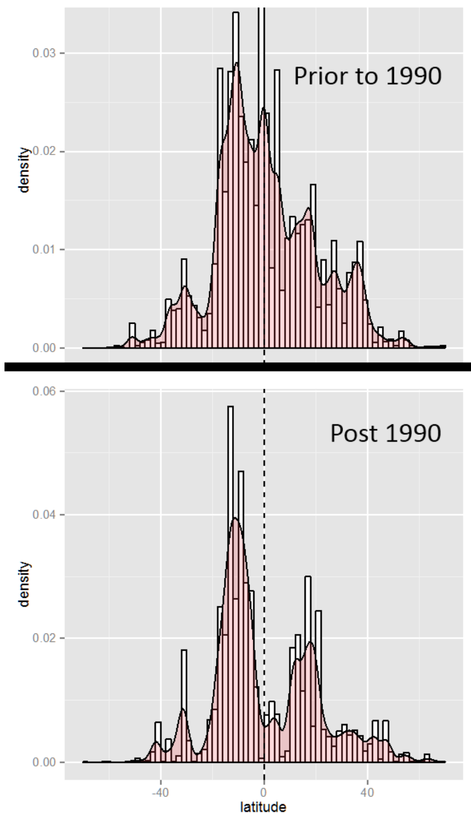
Рисунок 3.4 - Зміщення видів від екватору
