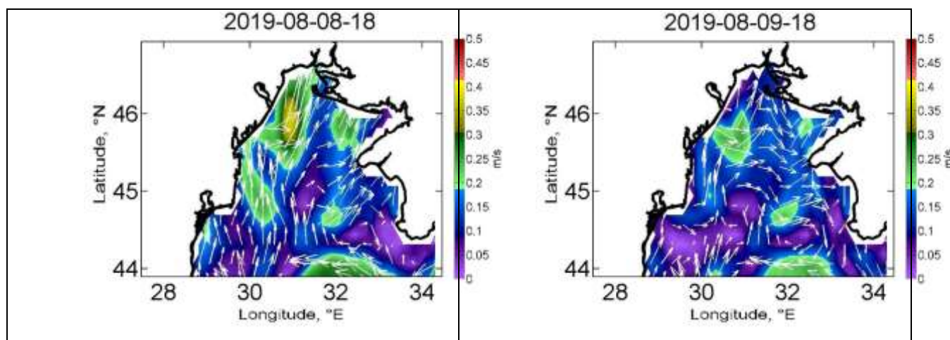
Рисунок 5.5, аркуш 2
