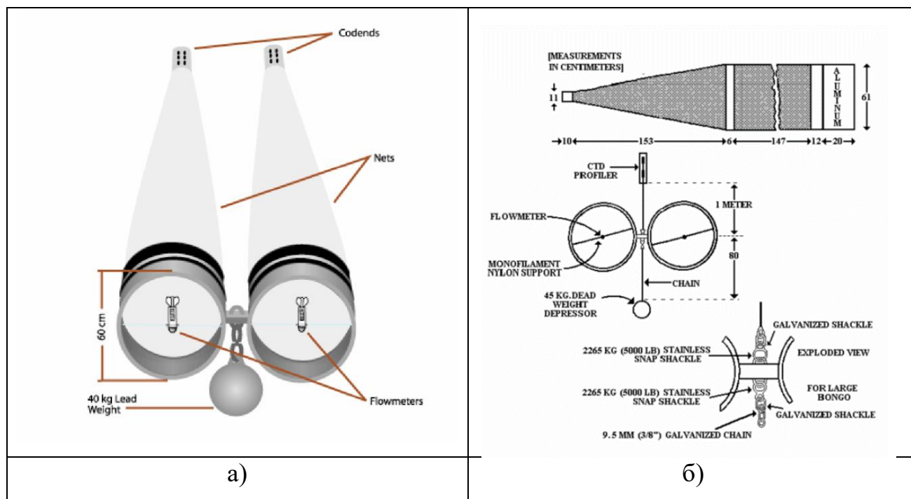
Рисунок 2.4 – Сітка Бонго (NOAA Fisheries Protocols for Ichthyoplankton Surveys, 2003): а) – вимірювач швидкості потоку встановлений в центрі гирла; знімний блок свинцю вагою 40-45 кг прикріплений до центрального стрижня на рамі, б) – схема колектору Бонго з відповідними розмірами (В).
