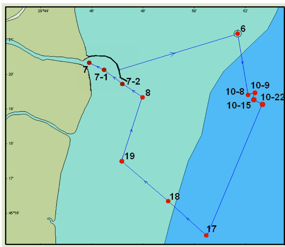
Рисунок 2.1 – Схема станцій моніторингу в районі дельти Дунаю у травні 2019 року
