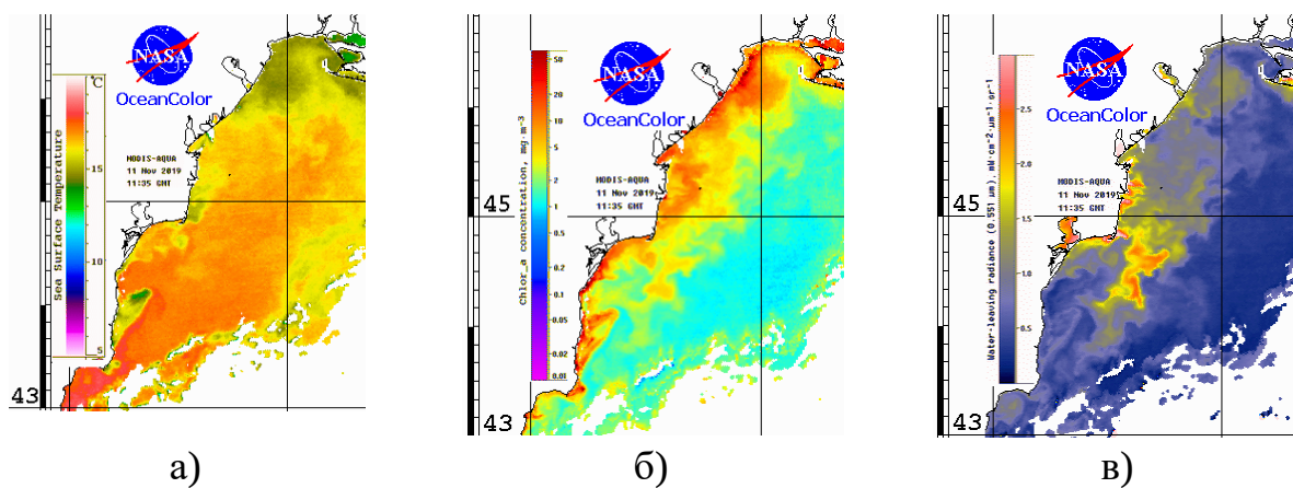
Рисунок 2.8 – Розподіли характеристик просторової мінливості вод 11.11.2019 р. у поверхневому шарі ПЗЧ Чорного моря за даними супутника MODIS: а) температура; б) хлорофіл-А; в) довгохвильове випромінювання.
