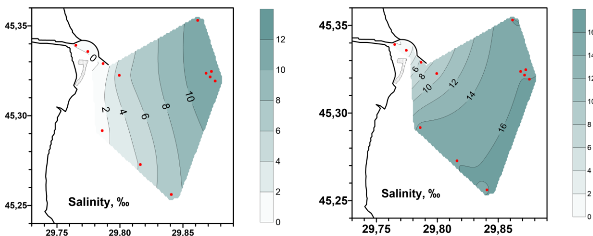
Рисунок 2.6 – Розподіл солоності на полігоні «Дунайський», травень 2019 р.: а) у поверхневому шарі; б) у придонному шарі.
