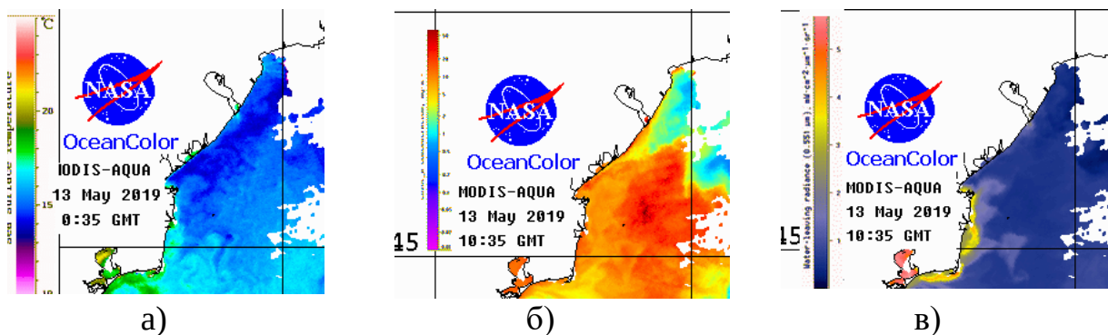
Рисунок 2.3 – Розподіли характеристик просторової мінливості вод 13.05.2019 р. у поверхневому шарі ПЗЧ Чорного моря за даними супутника
