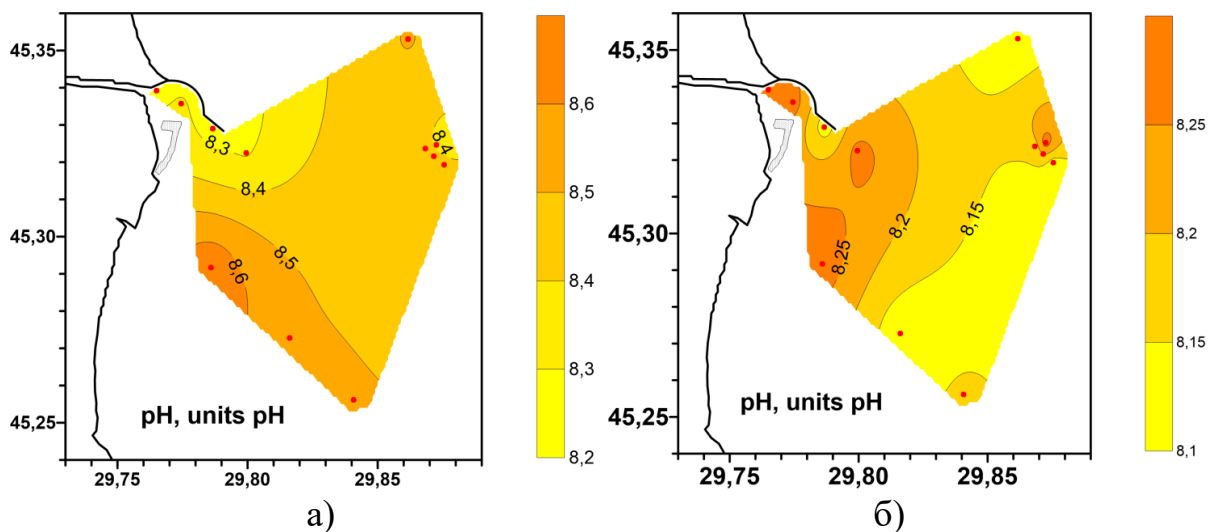
Рисунок 2.16 – Просторовий розподіл рН (од. рН) у морській частині дельти Дунаю у травні 2019 р.: а) у поверхневому шарі; б) у придонному шарі.
