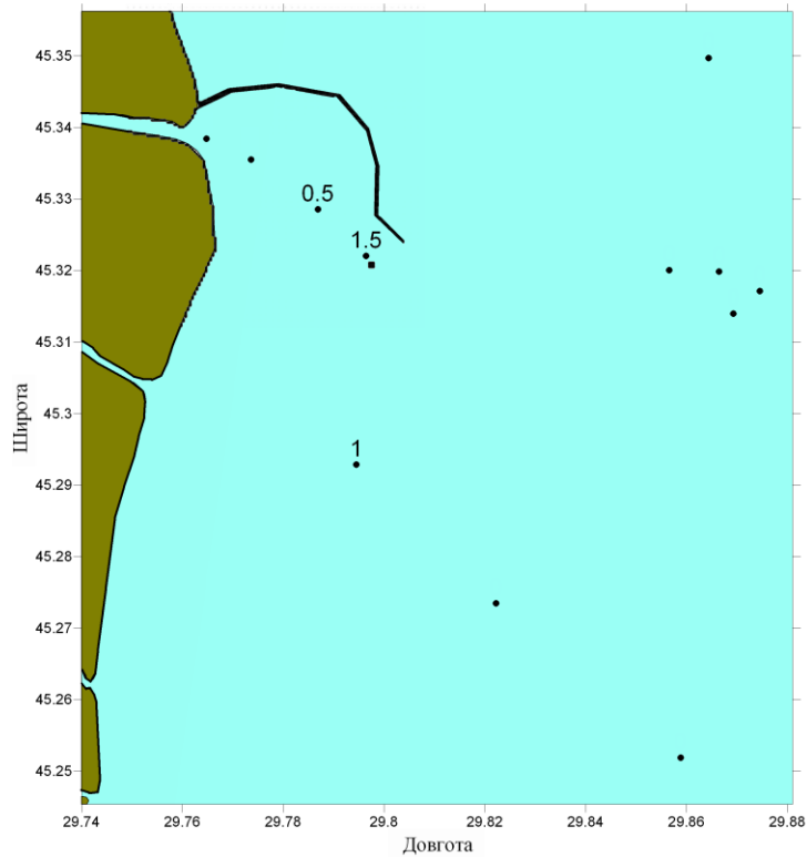
Рисунок 1.4 – Просторовий розподіл зон вторинного замулення донної поверхні моря в Дунайському районі ПЗЧМ (а), розподіл товщини намулку (мм) на придонному шарі відкладень (б) на Дунайському полігоні, 11.08.2020 р.
