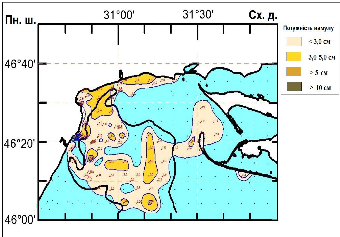
Рисунок 1.3–Просторовий розподіл зон вторинного замулення донної поверхні моря в Дніпро-Бузькому районі ПЗЧМ
