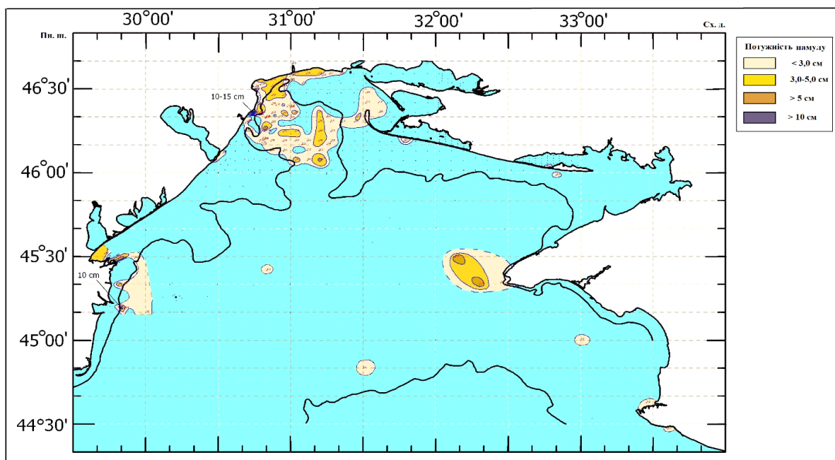
Рисунок 1.5 – Просторовий розподіл зон вторинного замулення донної поверхні моря на північно-західному шельфі Чорного моря
