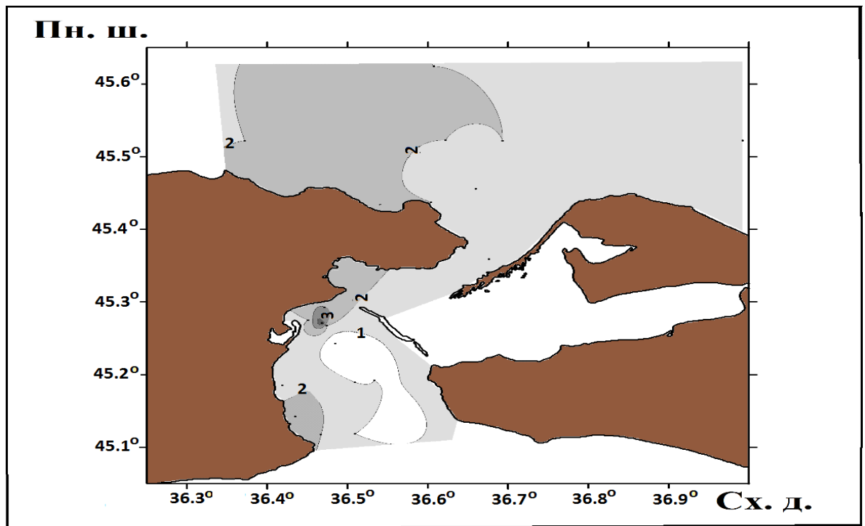
Рисунок 1.6 – Потужність шару (см) реседиментації донних відкладень в Керченській протоці в грудні 2009р.
