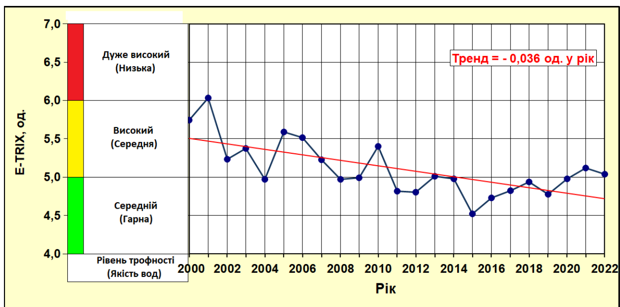
Рисунок 3.3 – Багаторічна мінливість тріфності і якості прибережних вод Одеського регіону ПЗШ ЧМ за показником TRIX
