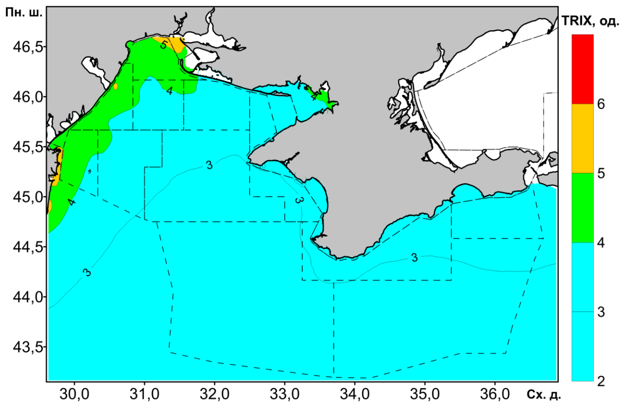
Рисунок 3.6 – Середньорічний просторовий розподіл значень показника TRIX в межах виключної морської економічної зони України у 2022 р.
