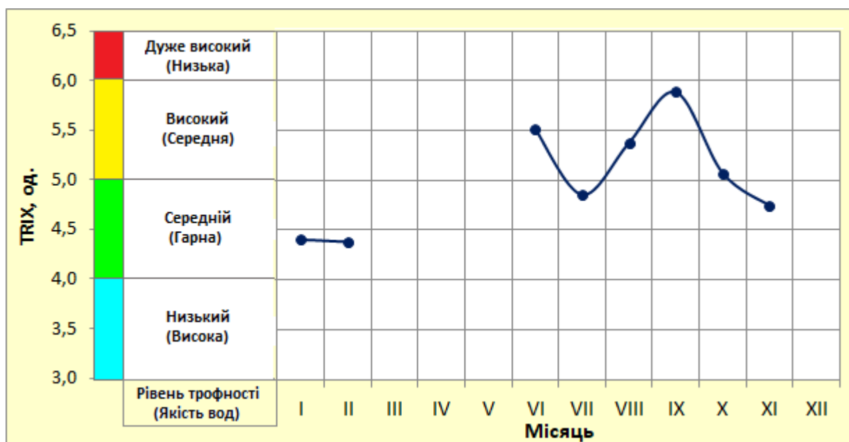
Рисунок 3.2 – Річний хід середніх місячних значень показника трофності TRIX прибережних вод м. Одеси у 2022 р.
