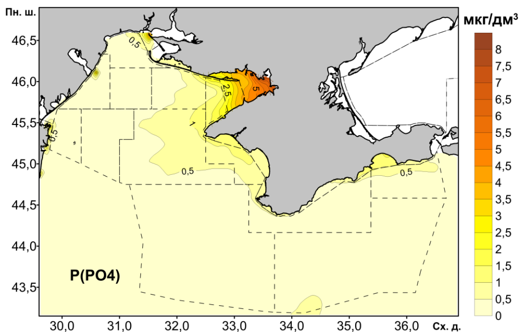
Рисунок 1.26 – Просторовий розподіл фосфору фосфатного в поверхневому шарі вод в межах виключної морської економічної зони України
