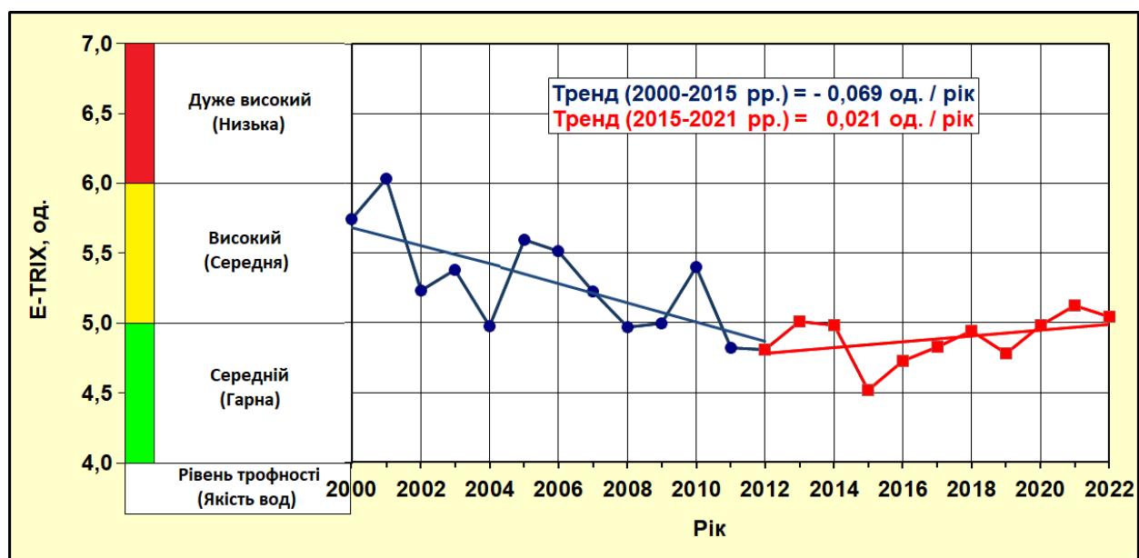
Рисунок 3.4 – Багаторічна мінливість тріфності і якості прибережних вод водного масиву CW5 Одеського регіону за показником TRIX
