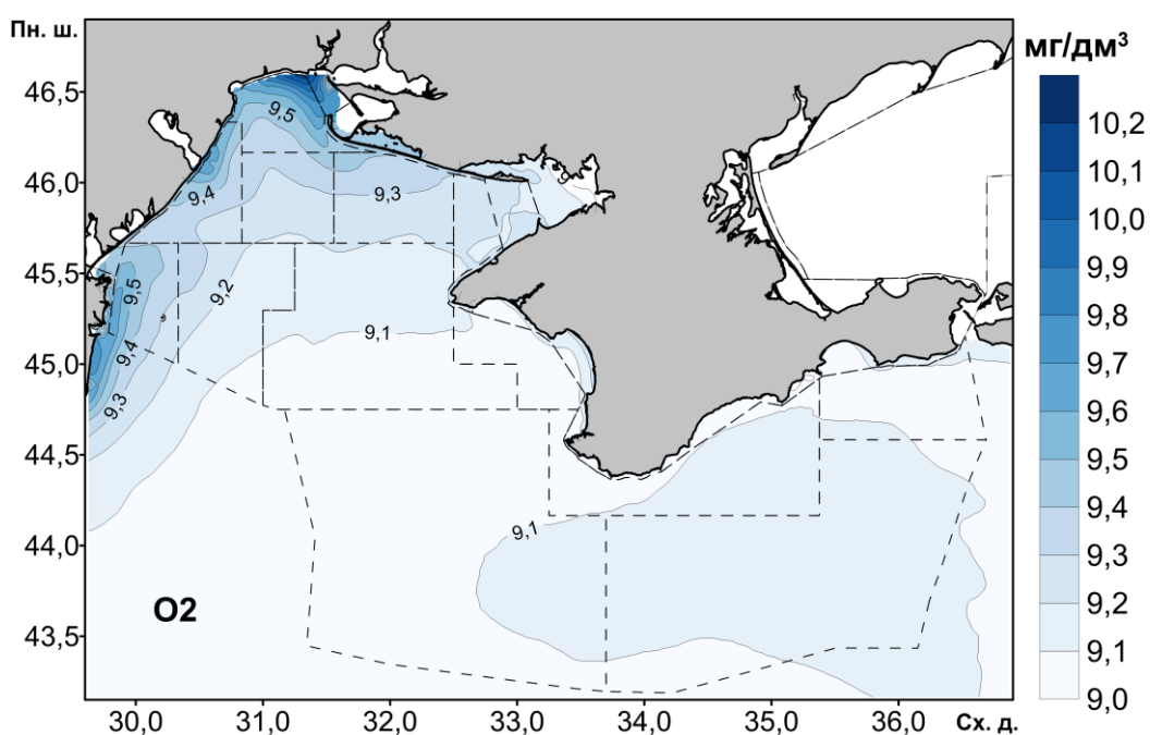
Рисунок 1.21 – Середньорічний поверхневий просторовий розподіл вмісту абсолютного кисню в межах виключної морської економічної зони України
