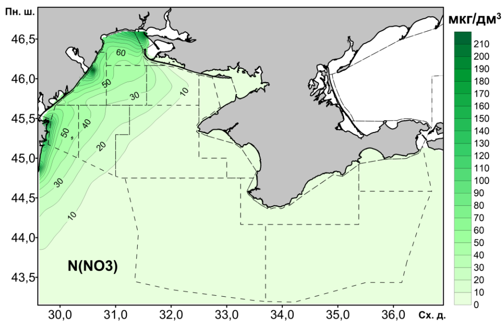
Рисунок 1.27 – Просторовий розподіл азоту нітратного в поверхневому шарі вод в межах виключної морської економічної зони України
