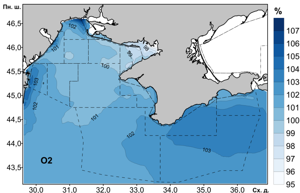
Рисунок 1.22 – Середньорічний поверхневий просторовий розподіл вмісту відносного кисню в межах виключної морської економічної зони України
