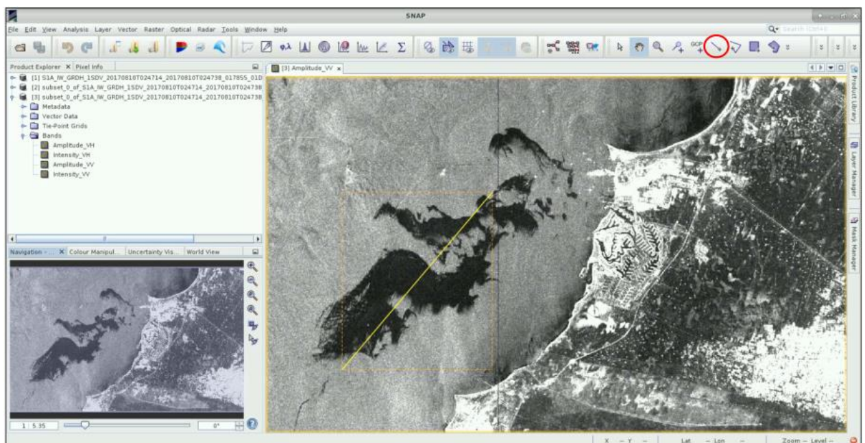
Рисунок А.9 – Лінія через розлив нафти
